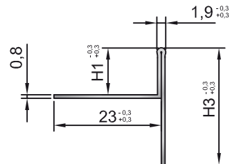
Querschnitt hinten
