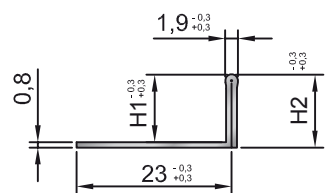
Querschnitt vorn
